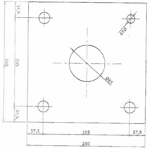
VISTA SUPERIOR DA SAPATA ESC.: 1 / 04
